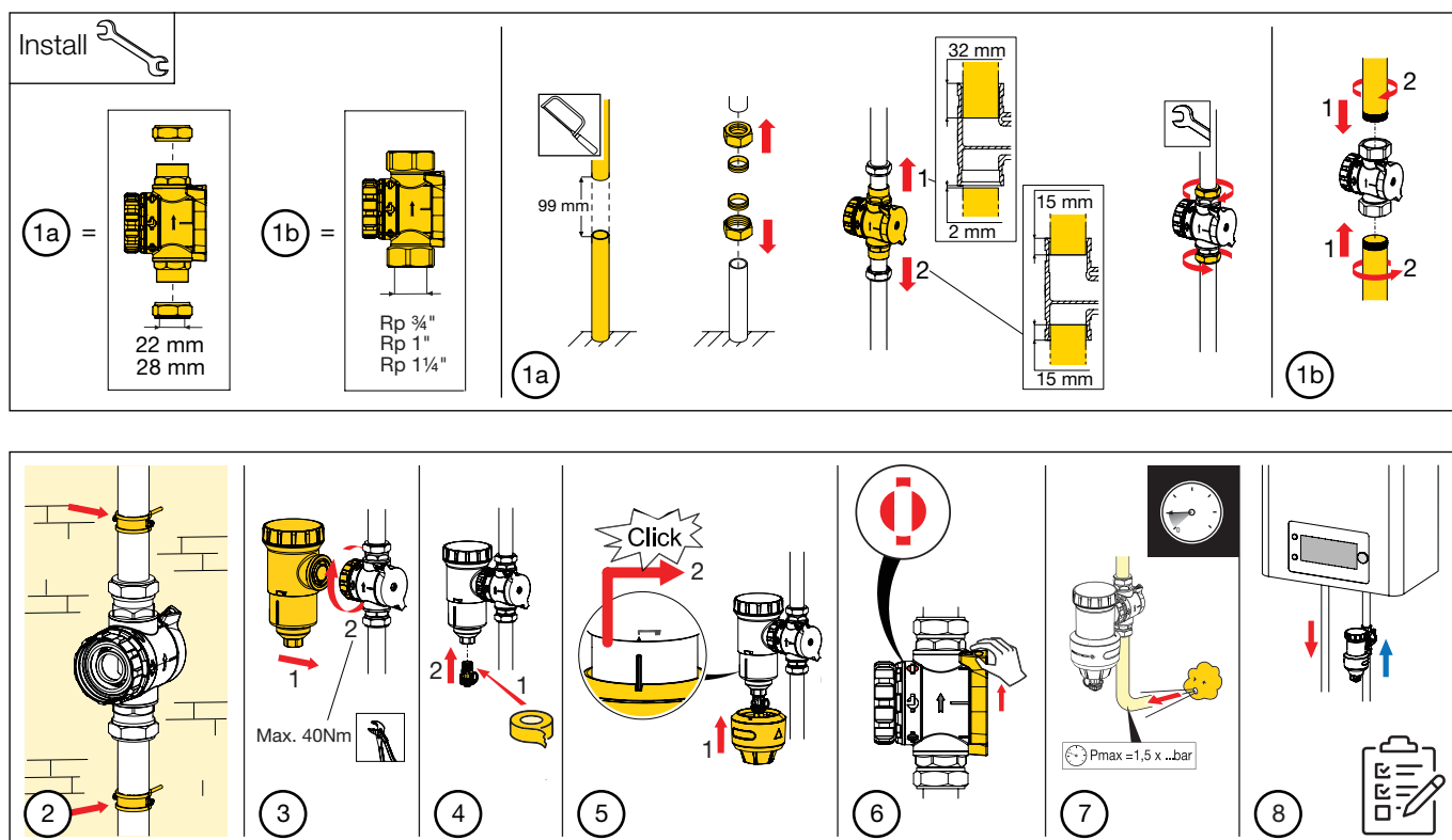
Figura 8: Installazione
