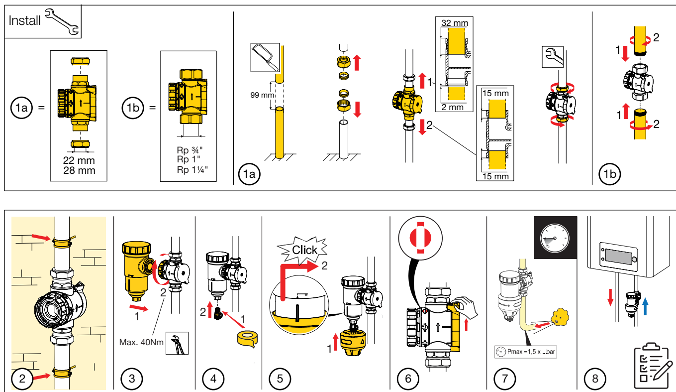
Abbildung 8: Installation
