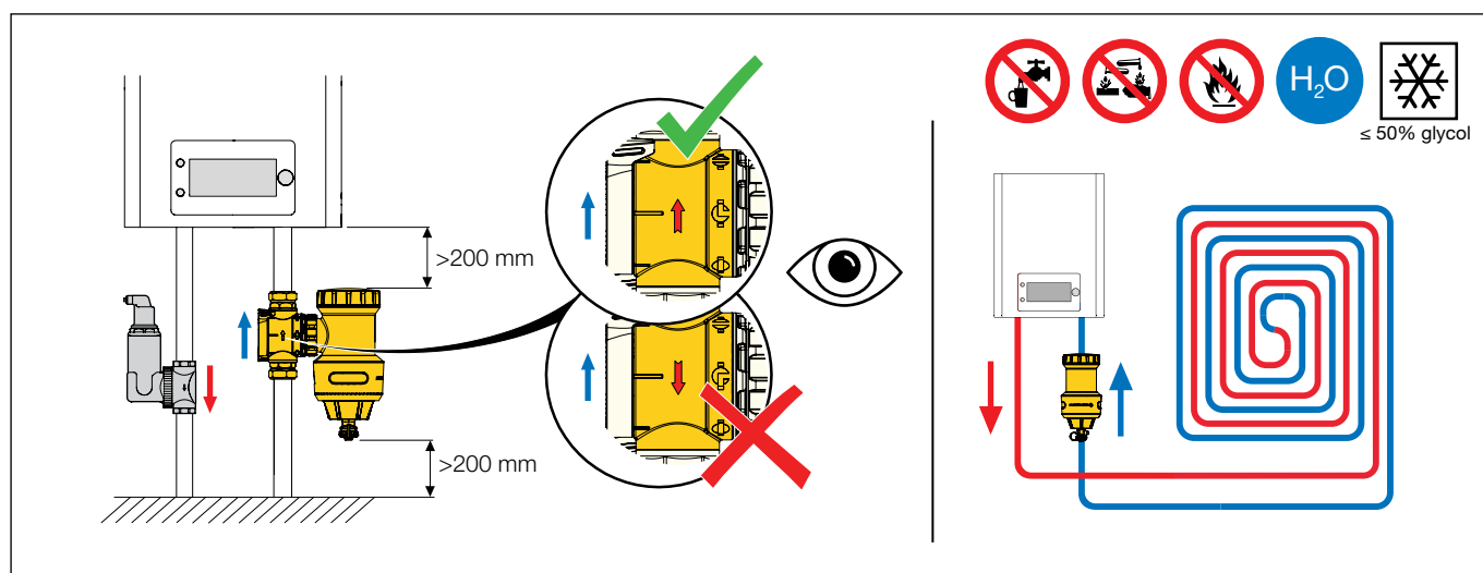
Figure 7: Positionnement
